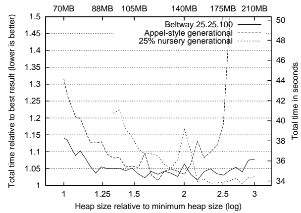
(f) pseudobjb
