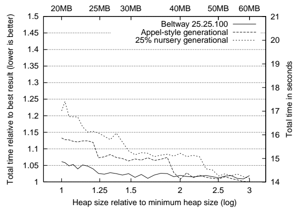
(e) _228_jack
